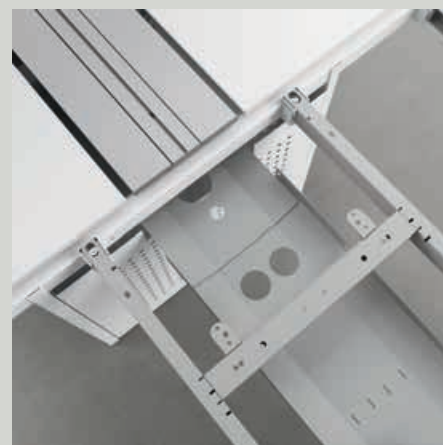
Prolunga in lamiera per canale passacavi per bench Sheet metal link-piece for bench cable duct
